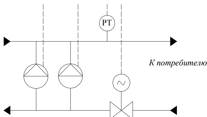
Рис. 1.2П. Гидромеханическая схема включения клапана
