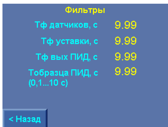
Рис. 10.20. Меню Фильтры
