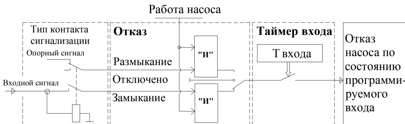
Рис.4.8. Программируемые входы
