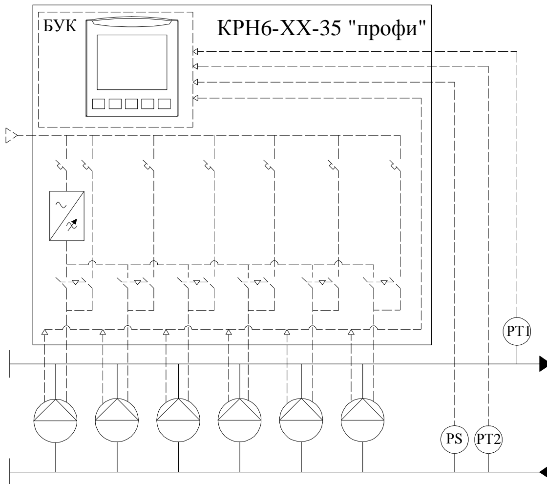
Рис. 2.2. Структурная схема установки повышения давления из 6 насосов, регулируемых КРН6- 35 «профи»
