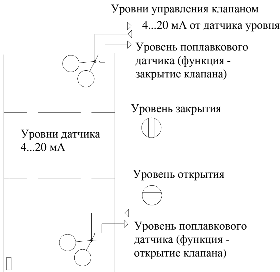
Рис. 8.2П. Функциональная схема управления клапаном подпитки
