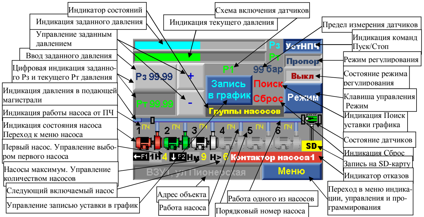
Рис.7.1. Главное меню
