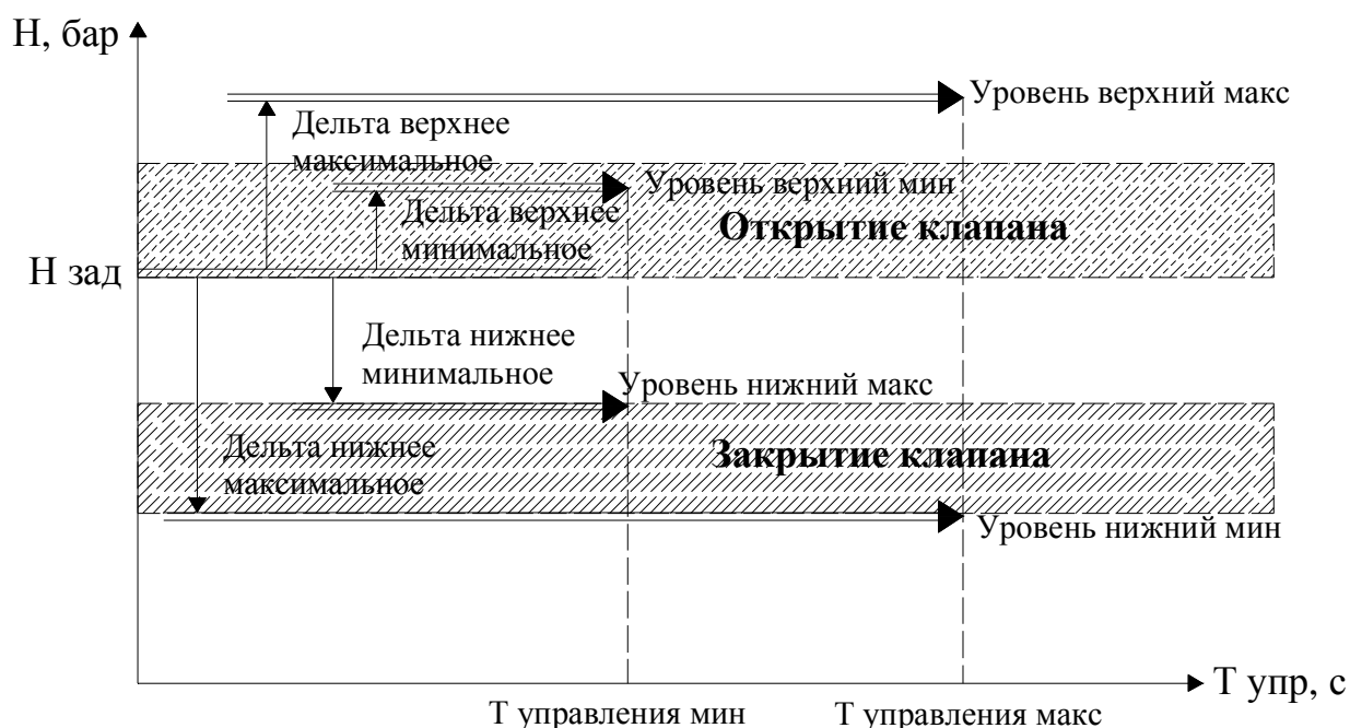
Рис. 2.2П. Алгоритмическая схема управления клапаном
