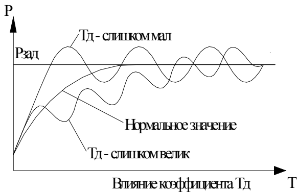
Рис.10.12. Влияние коэффициентов ПИД - регулятора на параметры переходных процессов
