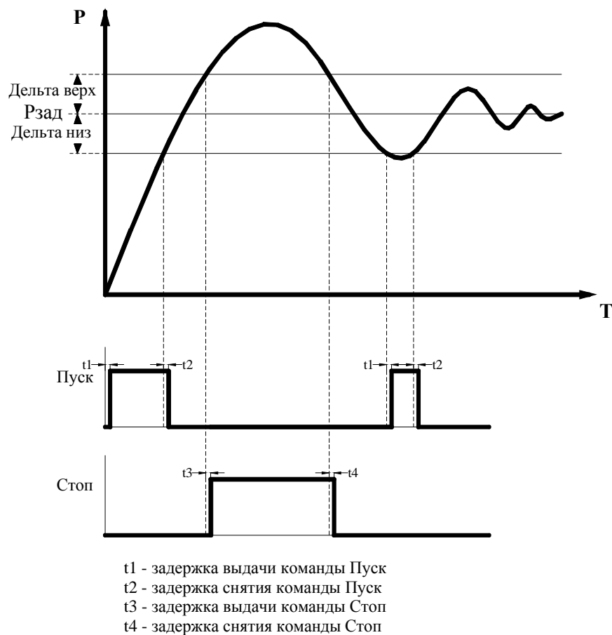
Рис. 4.1. Формирование команд ПУСК/СТОП
