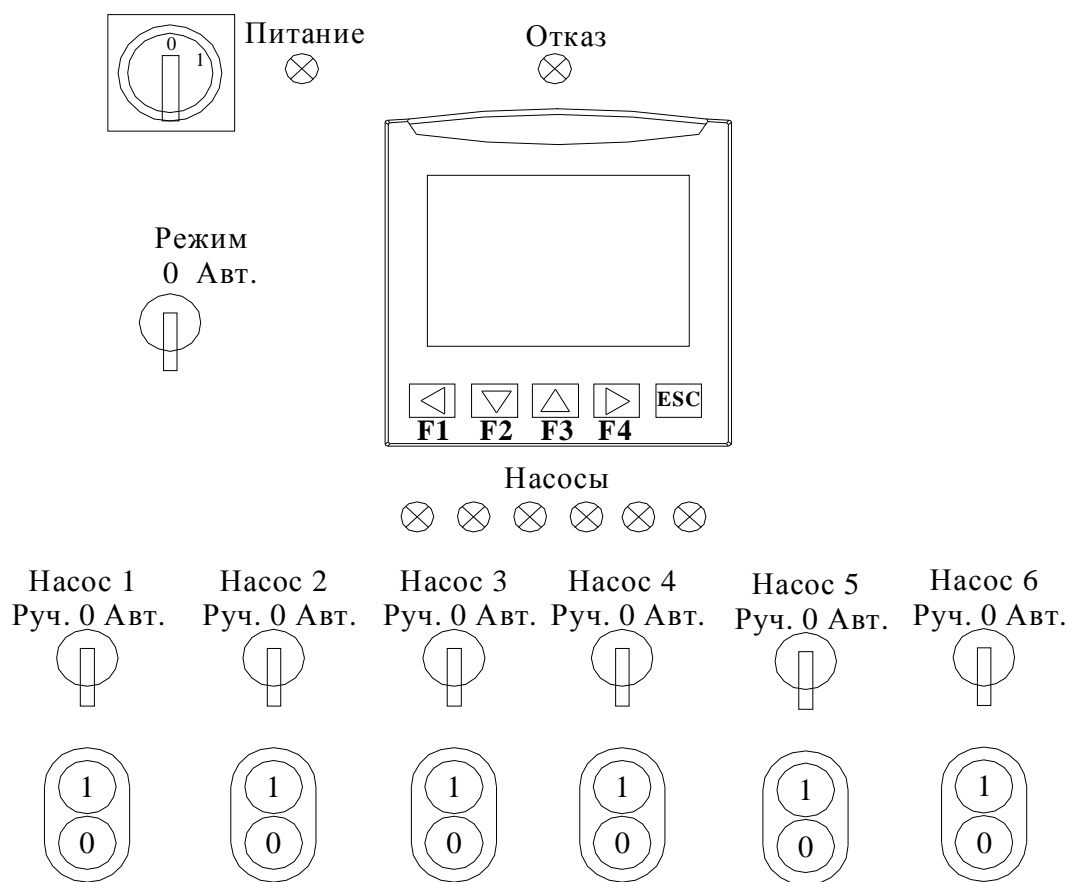
Рис. 6.1. Система управления и индикации КРН серии 35 «профи»
