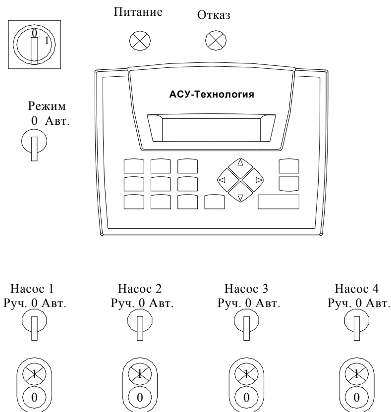
Рис. 4.1. Панель управления и индикации ШУН
