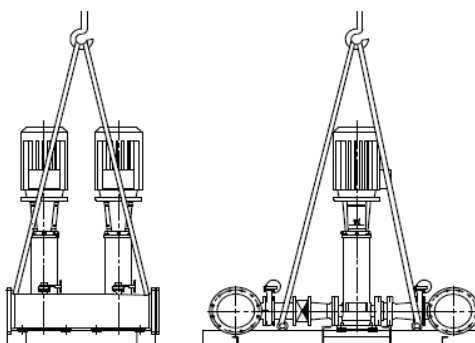
Рис. 7. Правильный подъём установок Hydro AT(П)
