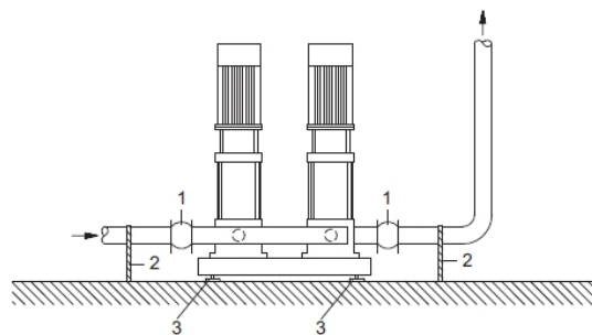
Рис. 8. Положение вибровставок, опор для труб и вибрационных опор
