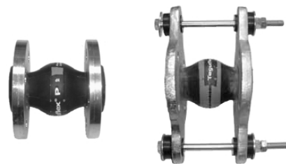
Рис. 9. Вибровставки с резиновыми прокладками без ограничительных стяжек и с ними
