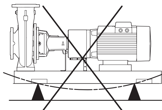
Рис. 25 Неправильный фундамент
