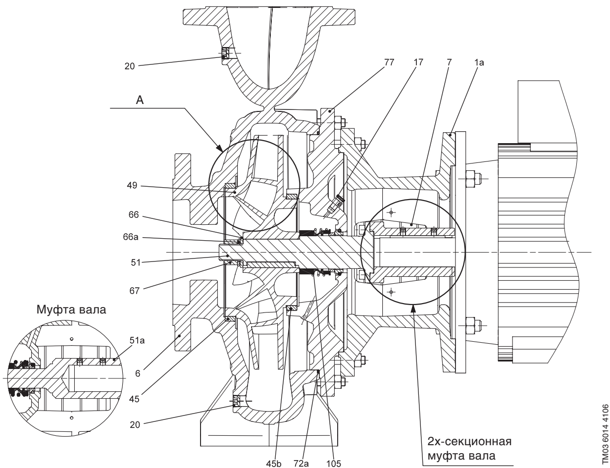
Рис. 3 Насос NB в разрезе
