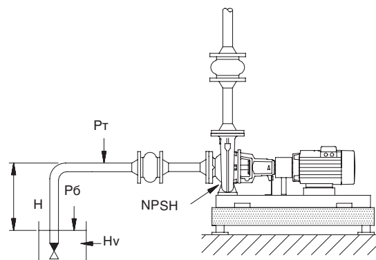
Рис. 22 Схема открытой системы с насосом NK
