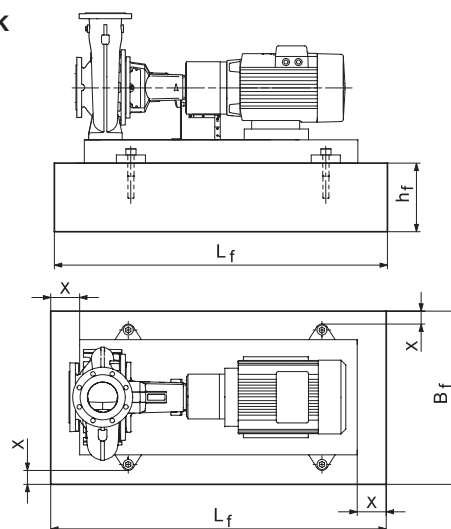
Рис. 23 Фундамент
