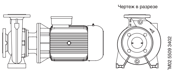
Рис. 5 Насос NB, исполнение А
