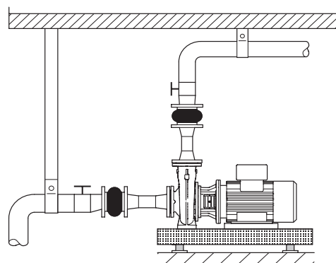
Рис. 29 Монтаж трубопровода
