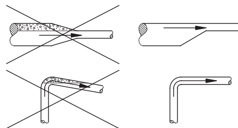
Рис. 28 Трубопровод
