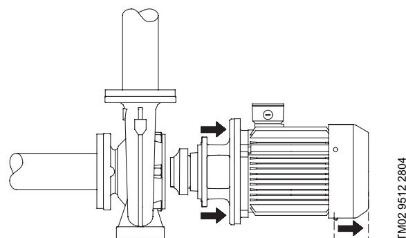
Рис. 1 Демонтаж электродвигателя насоса NB
