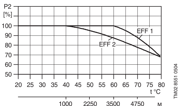
Рис. 19 Зависимость мощности электродвигателя P2 от температуры/высоты размещения над уровнем моря
