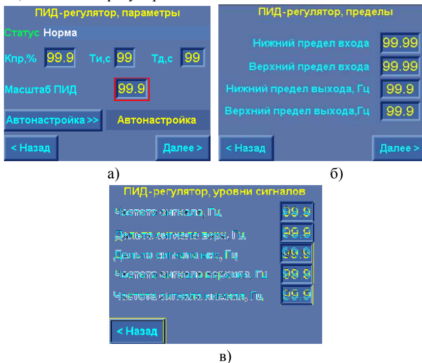
Рис. 10.14. Меню ПИД - регулятор
