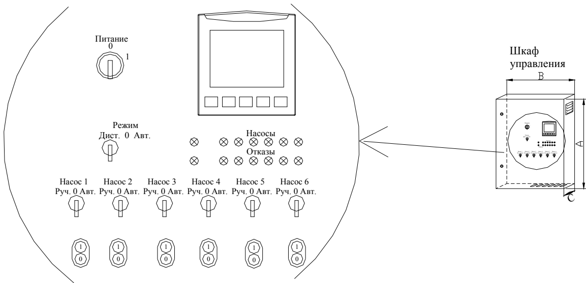
Внешний вид КРН в напольном исполнении
