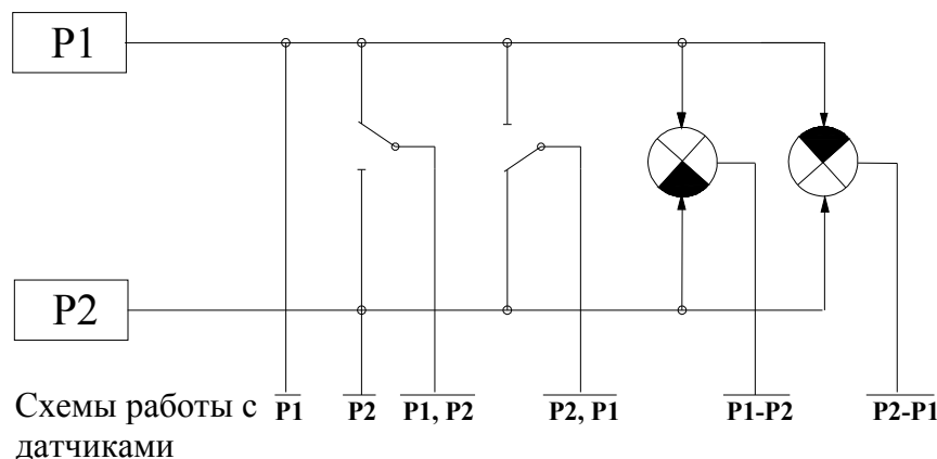
Рис.4.4. Схема работы с аналоговыми датчиками давления
