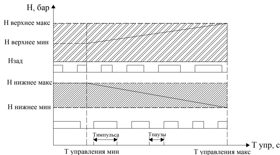
Рис. 7.2П. Изменение длительности управляющего импульса в нижнем и верхнем диапазонах
