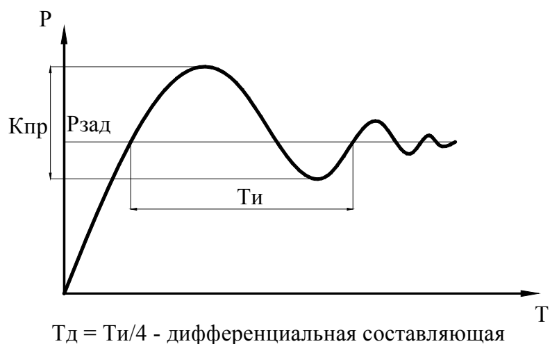
Рис. 10.15. Значения параметров ПИД-регулятора
