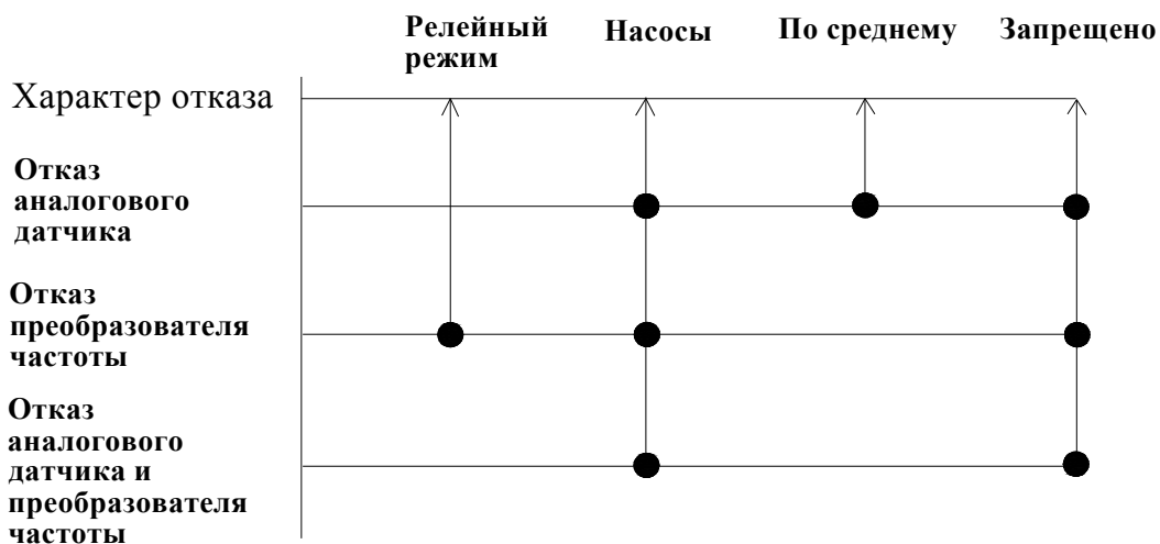
Рис.5.4. Схема перехода в режимы функционального резерва
