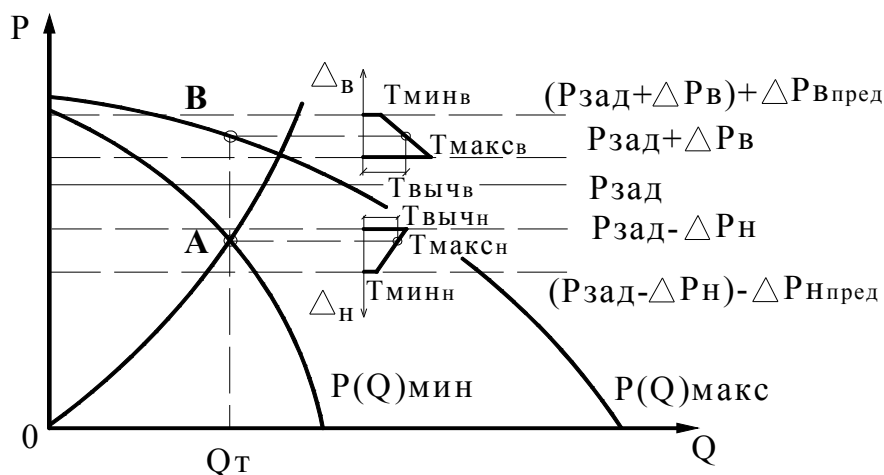
Рис. 4.7. Функция повышения устойчивости системы регулирования
