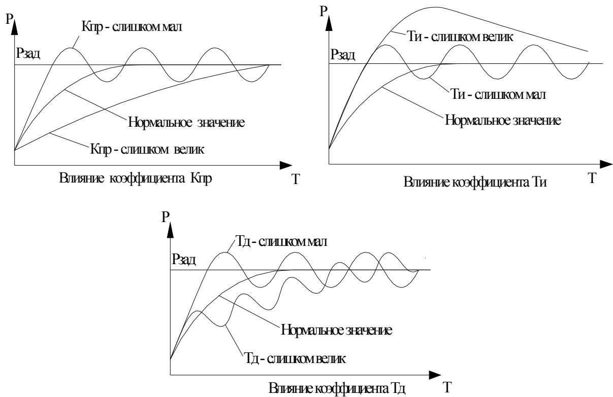
Рис.10.16. Влияние коэффициентов ПИД - регулятора на параметры переходных процессов
