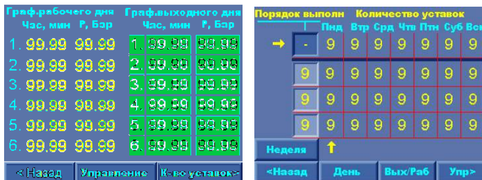
Рис. 10.18. Меню Графики давлений а) параметры графиков; б) количество уставок
