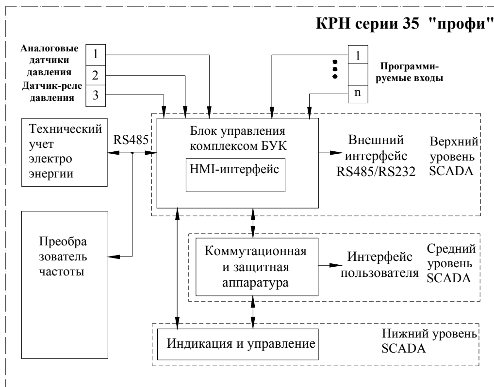
Рис.2.1. Структурная схема КРН серии 35 «профи»
