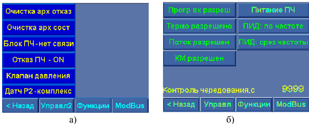
Рис. 5.1П. Меню Управление
