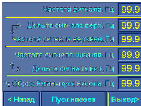
Рис. 9.6. Уровни сигналов ПИД
