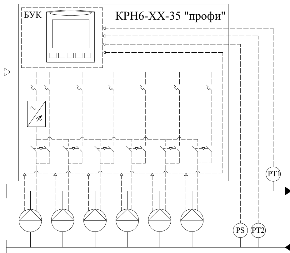
Рис. 2.2. Структурная схема установки повышения давления из 6 насосов, регулируемых КРН6-35 «профи»
