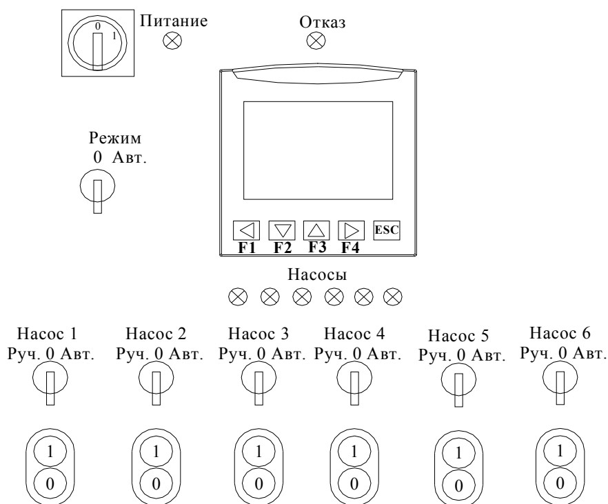
Рис. 6.1. Система управления и индикации КРН серии 35 «профи»
