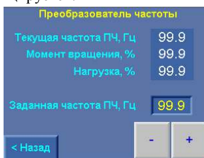
Рис. 9.4. Меню Индикации параметров ПЧ в режиме рампы
