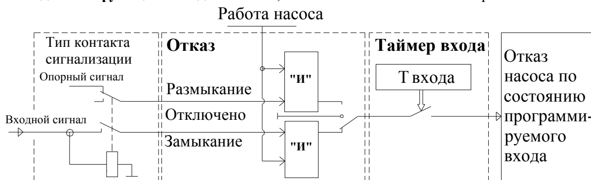
Рис.4.89. Программируемые входы
