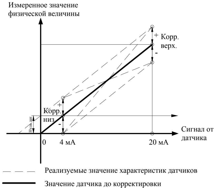
Рис.4.5. График коррекции характеристики датчика
