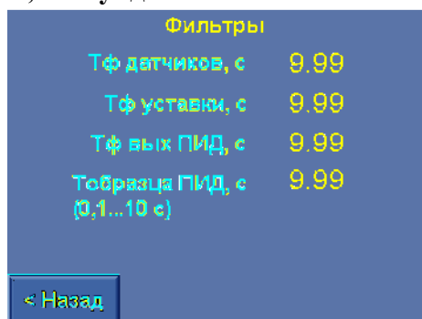
Рис. 10.24. Меню Фильтры
