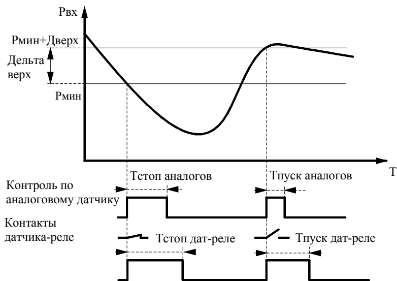
Рис.4.8. Формирование сигнала снижения давления во входной магистрали
