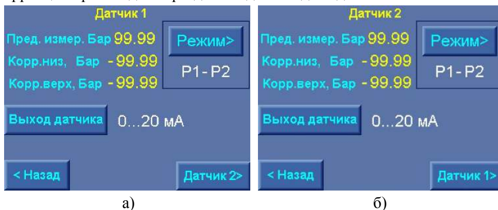
Рис.10.7. Меню «Датчики»
