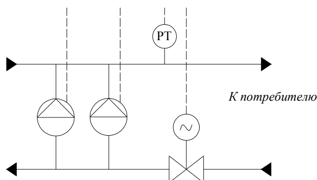
Рис. 1.2П. Гидромеханическая схема включения клапана
