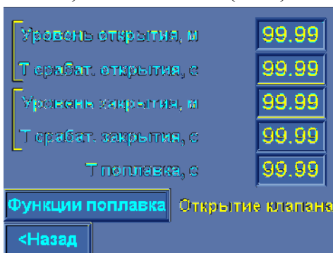
Рис. 9.2П. Меню Клапана подпитки
