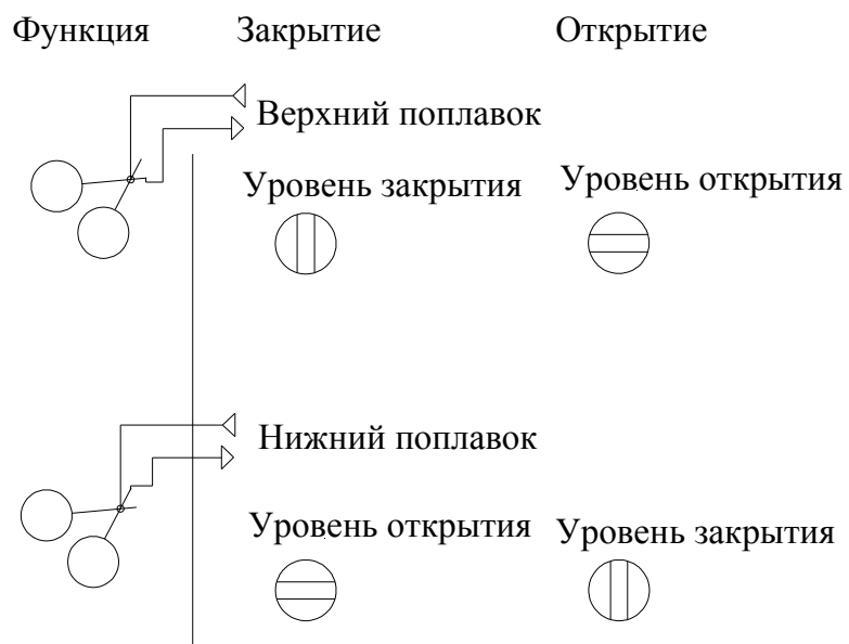
Рис. 10.2П. Функциональная схема управления клапаном подпитки по двум поплавковым датчикам
